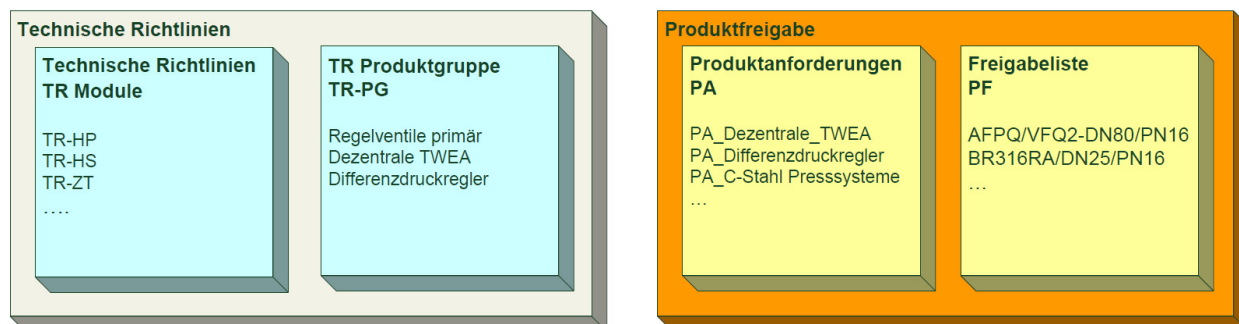
Abbildung 3: Zusammenhang Technische Richtlinien und Produktfreigabe
