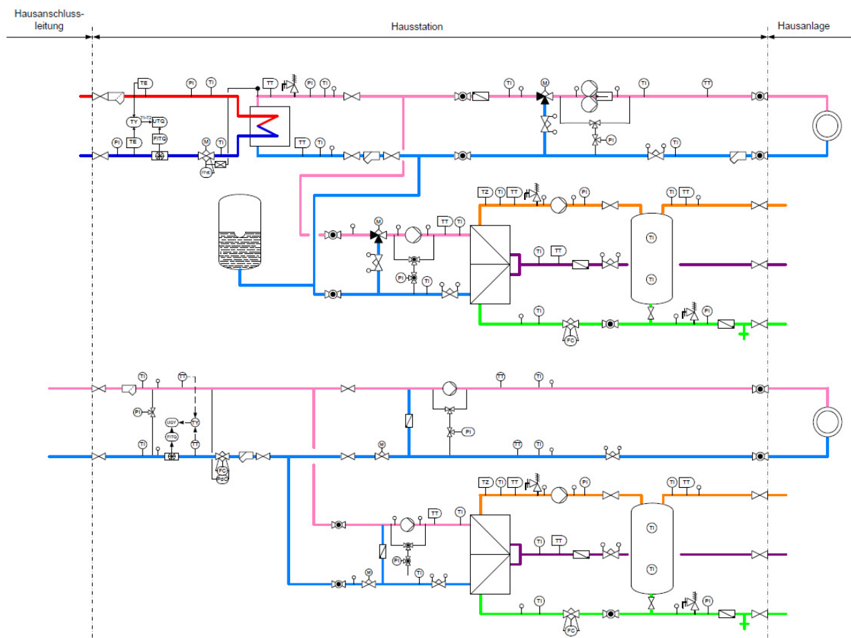
Abbildung 1: Definition Hausstation
