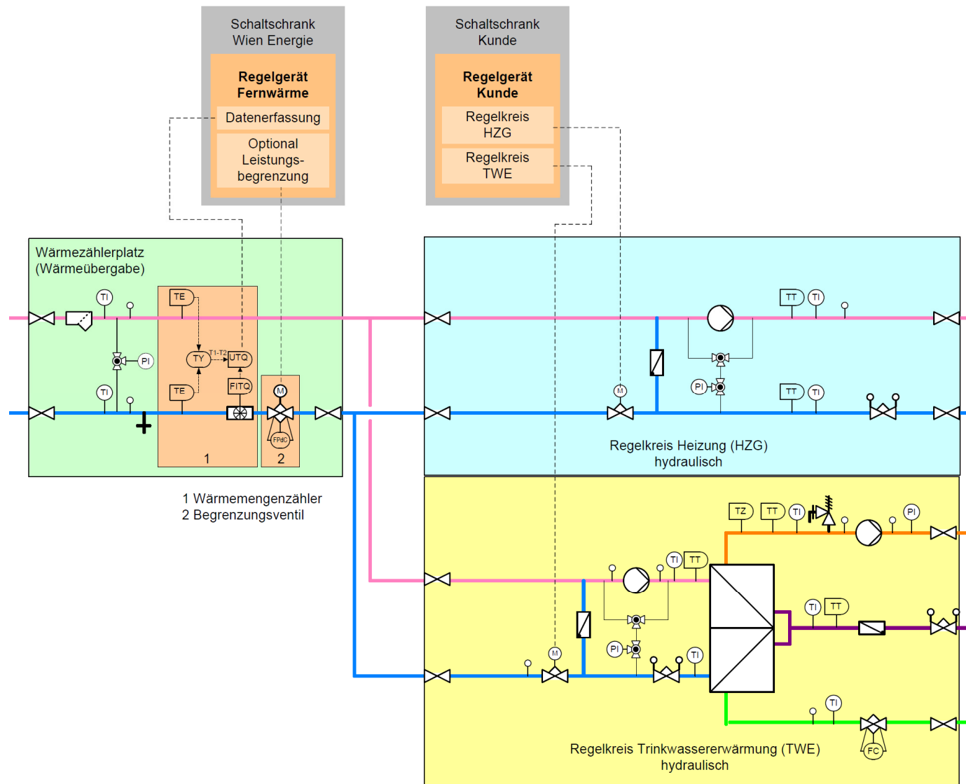
Abbildung 9: Fernwärmeregulation bei Versorgung aus dem Sekundärnetz bei kundeneigener Regelung
