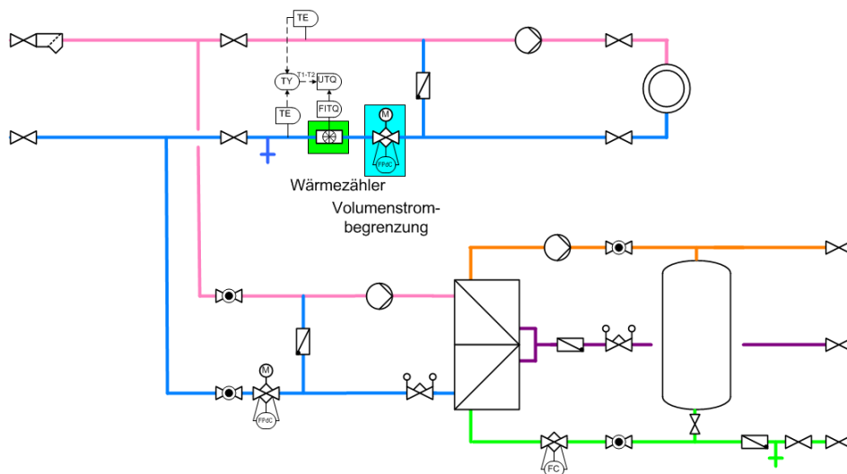
Abbildung 5: Rahmenvertrag, Positionierung Verrechnungszähler und Volumenstrombegrenzung
